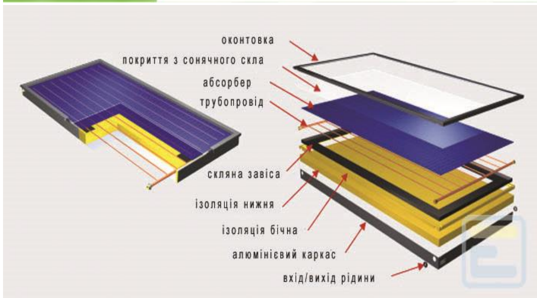
рисунок 2–Принцип дії сонячної батареї
