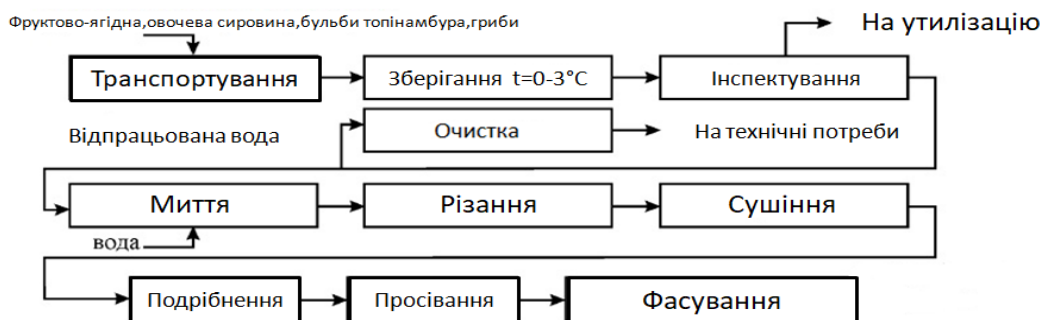
Принципова схема технологічного процесу виробництва фруктово-ягідних, грибних і порошоків з коренів бульб
