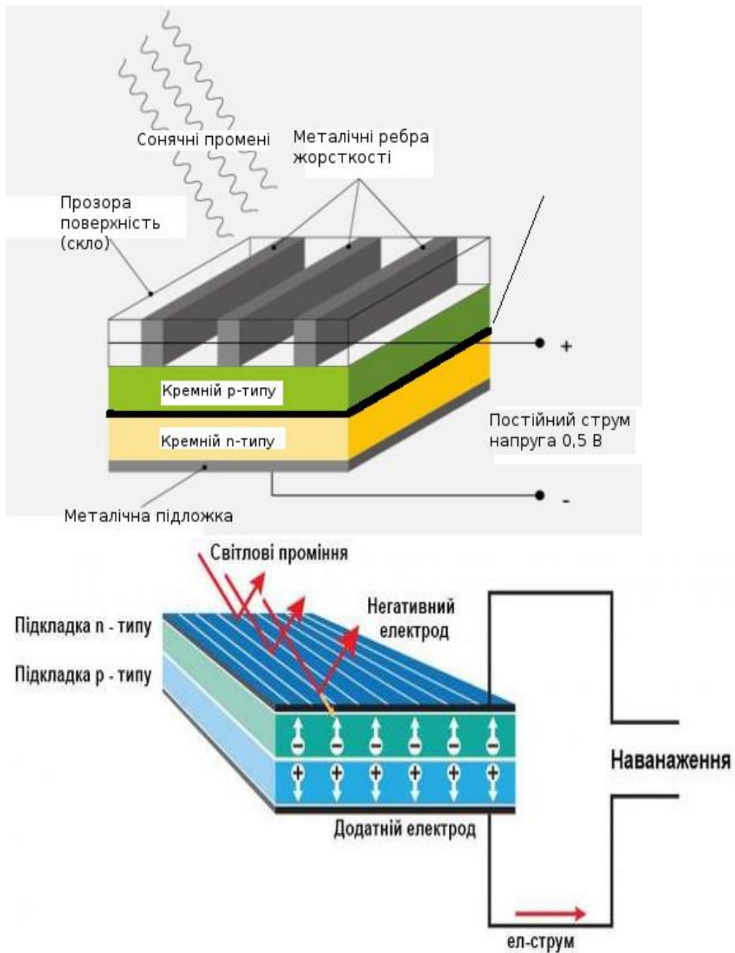
рисунок 1–Конструкція сонячної батареї
